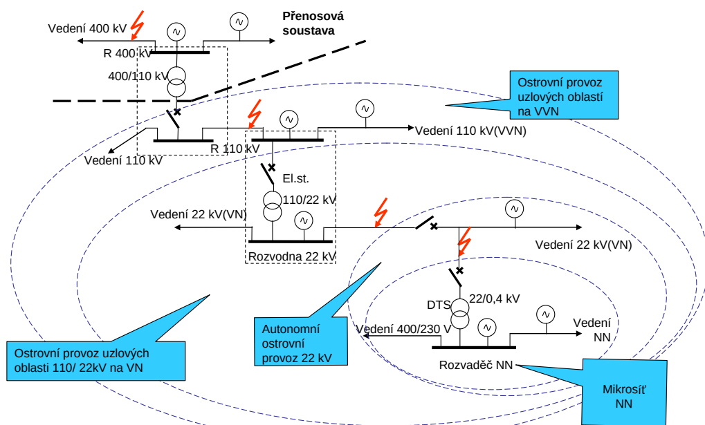
Obrázek 57 Možnosti ostrovního provozu v distribuční soustavě
