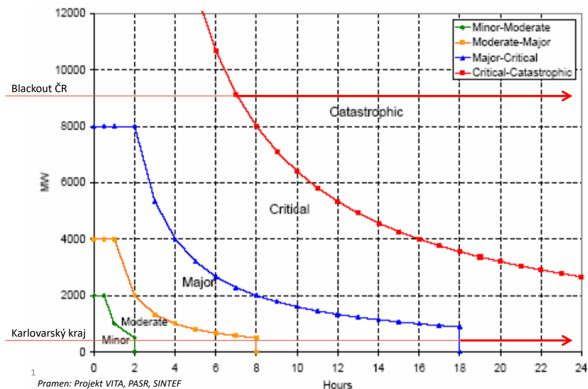
Obrázek 37 Kritičnost situace v závislosti na rozsahu a délce výpadku elektřiny
