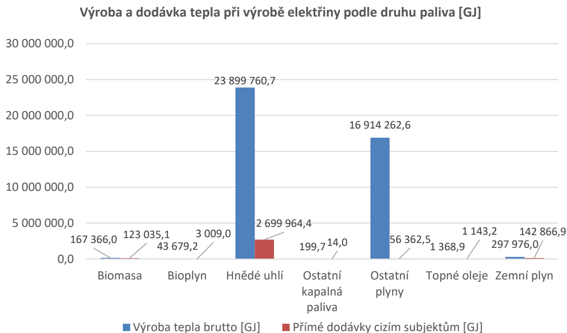
Graf 59 Balance výroby a dodávky tepla při výrobě elektřiny podle druhu paliva
