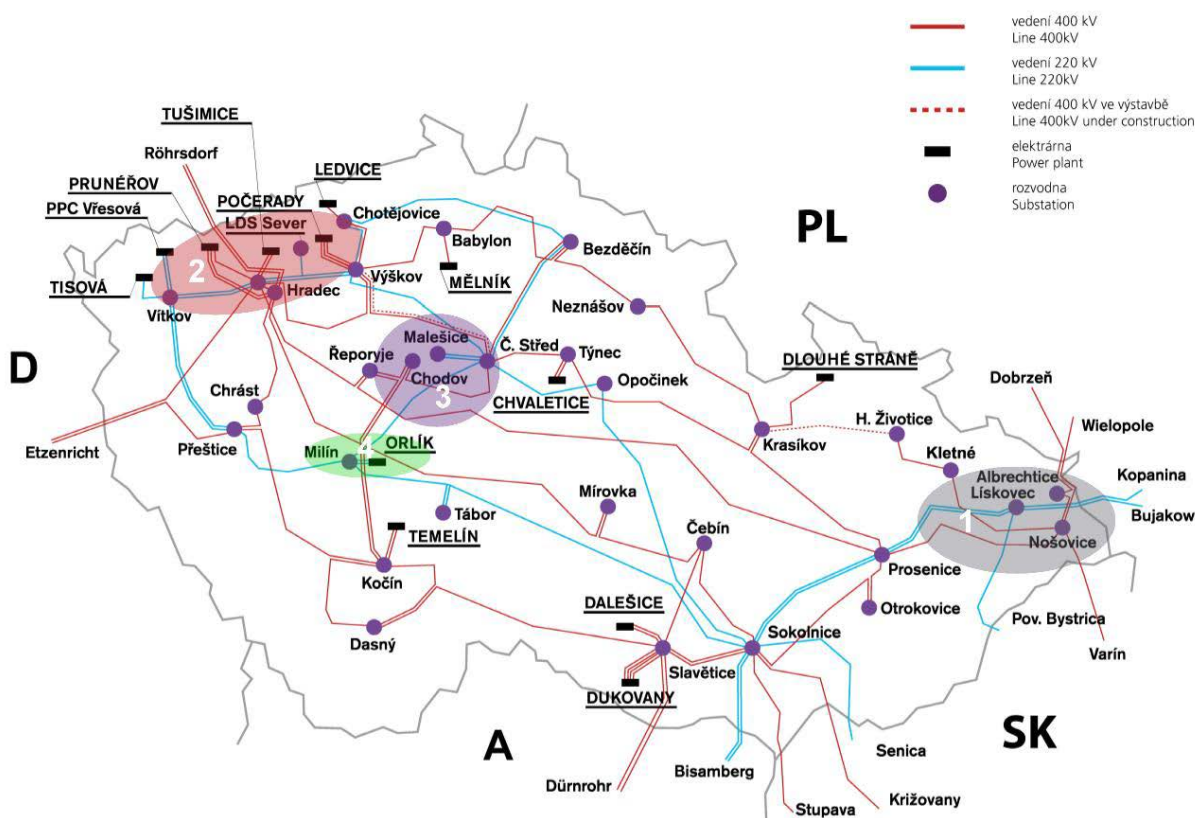
Obrázek 15 Rozvoj spotřeby a transformačních vazeb PS/DS
