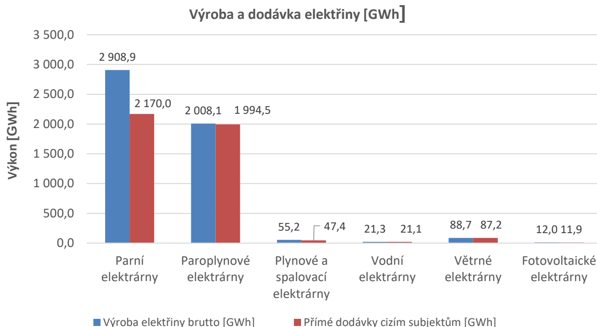
Graf 42 Výroba a dodávka elektřiny dle technologie elektrárny
