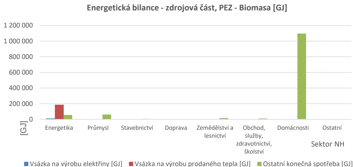
Graf 34 Energetická bilance-zdrojová část, PEZ – Biomasa, rok 2014
