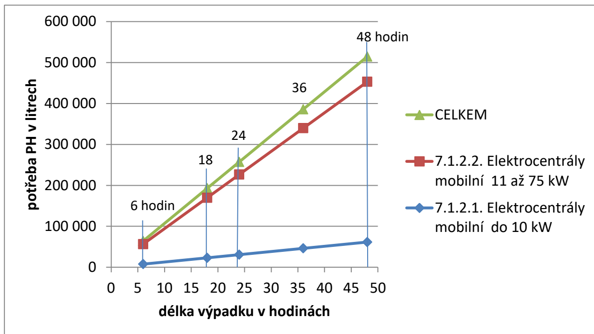
Obrázek 35 Potřeba pohonných hmot pro elektrocentrály požadované v systému ARGIS
