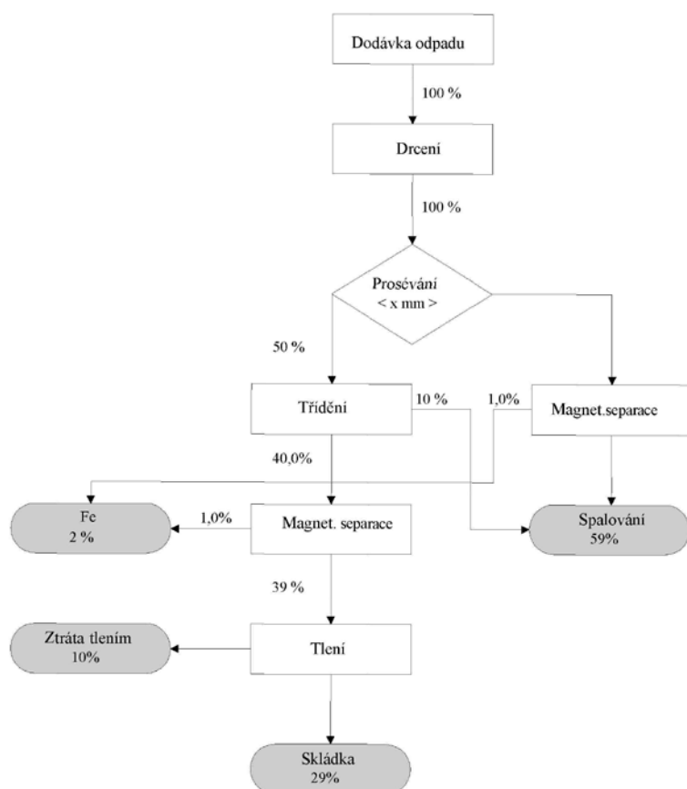
Obrázek 29 Schéma mechanicko-biologické úpravy odpadů v kombinaci se zařízením na spalování (energetického využívání) vysokovýhřevného odpadu.
