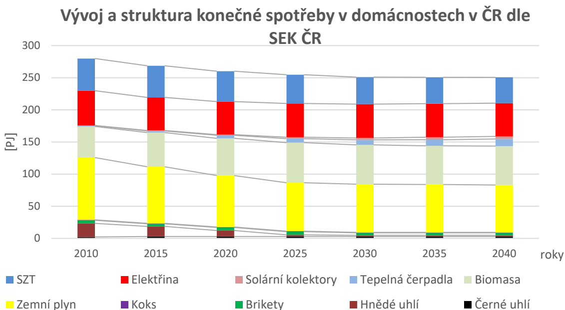
Graf 78 Vývoj a struktura konečné spotřeby energie v domácnostech ČR dle SEK ČR
