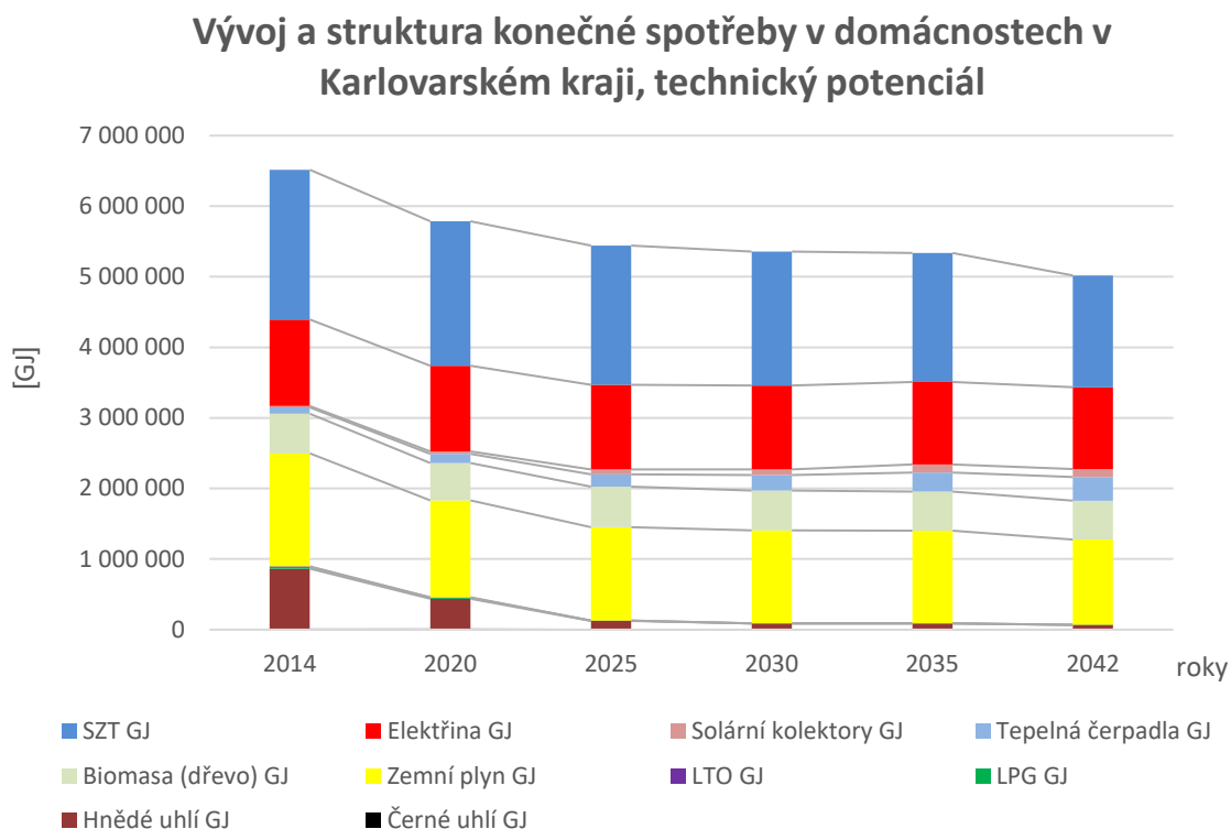
Graf 87 Vývoj a struktura konečné spotřeby v domácnostech v Karlovarském kraji, technický potenciál
