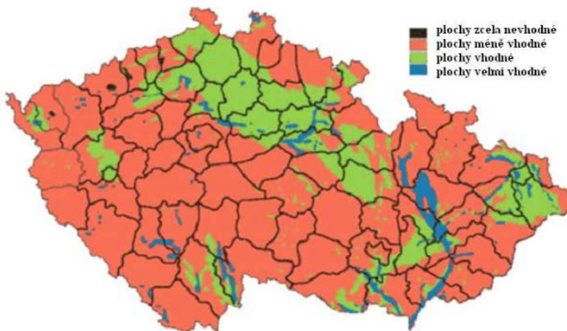
Obrázek 25 Potenciál geotermální energie v ČR
