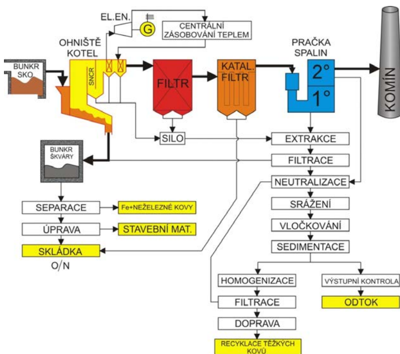
Obrázek 28 Schéma řazení jednotlivých technologií ZEVO
