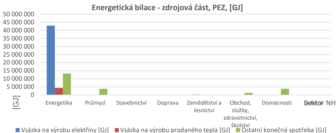
Graf 31 Energetická bilance-zdrojová část, PEZ společně pro všechny paliva, rok 2014
