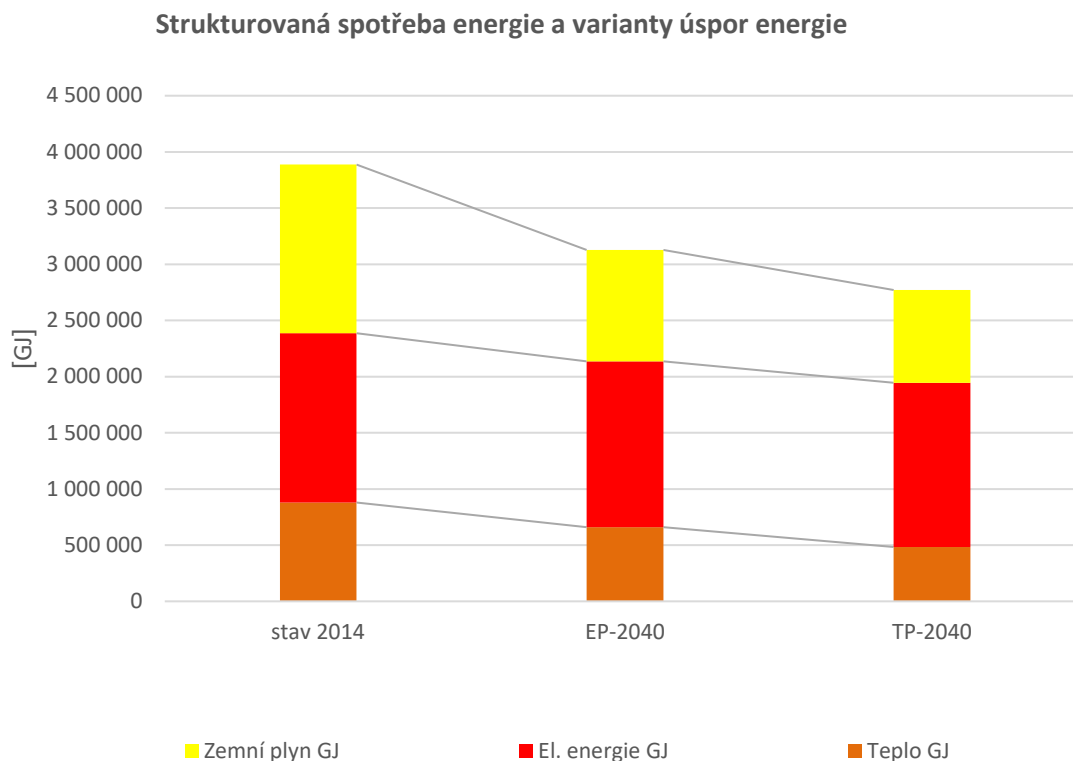
Graf 92 Strukturovaný přehled spotřeby energie ve veřejném sektoru a potenciál úspor pro varianty TP a EP oproti roku 2014
