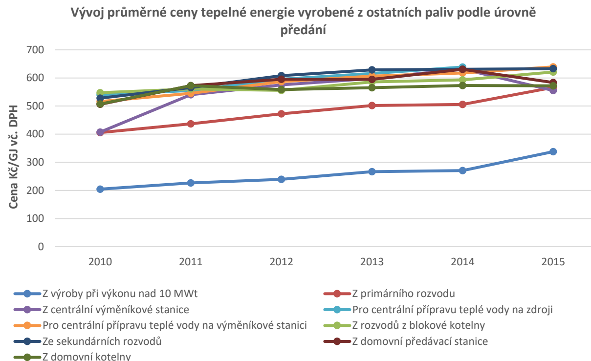
Graf 64 Vývoj průměrné ceny tepelné energie vyrobené z ostatních paliv podle úrovně předání, Karlovarský kraj
