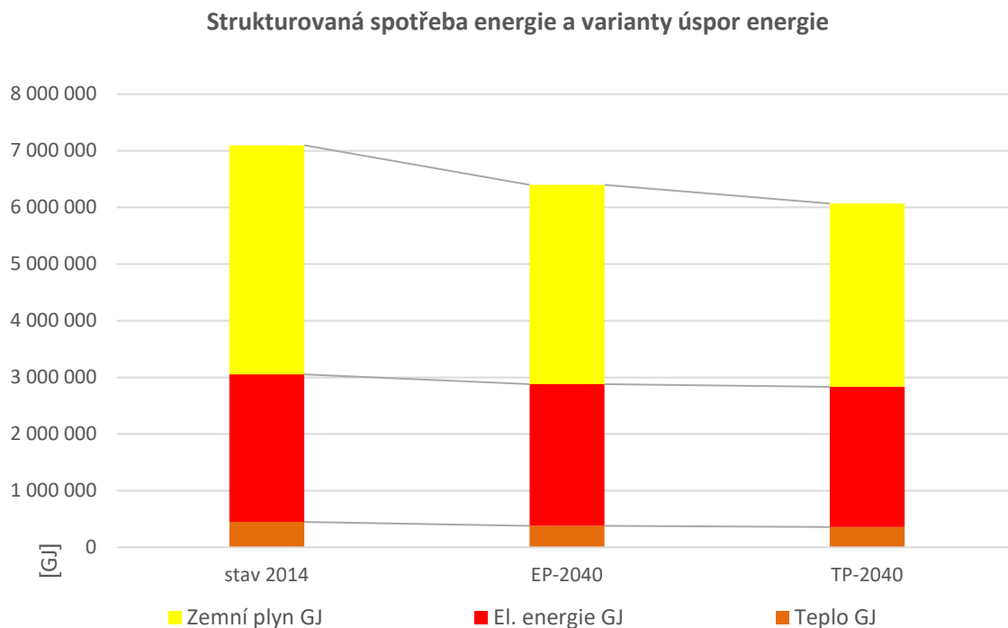
Graf 94 Strukturovaný přehled spotřeby energie v podnikatelském sektoru a potenciál úspor pro varianty TP a EP oproti roku 2014
