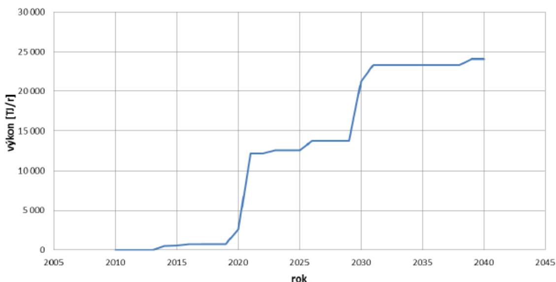
Graf 73 Vývoj výpadku dodávek tepla z tepláren
