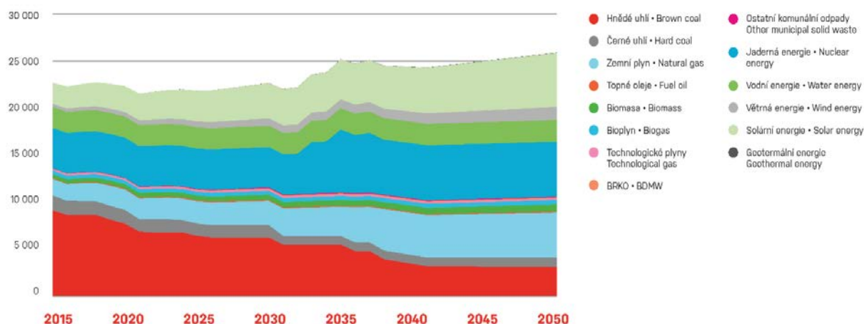
Graf 50 Predikce vývoje instalovaného výkonu v ES ČR v členění dle primárních zdrojů energie
