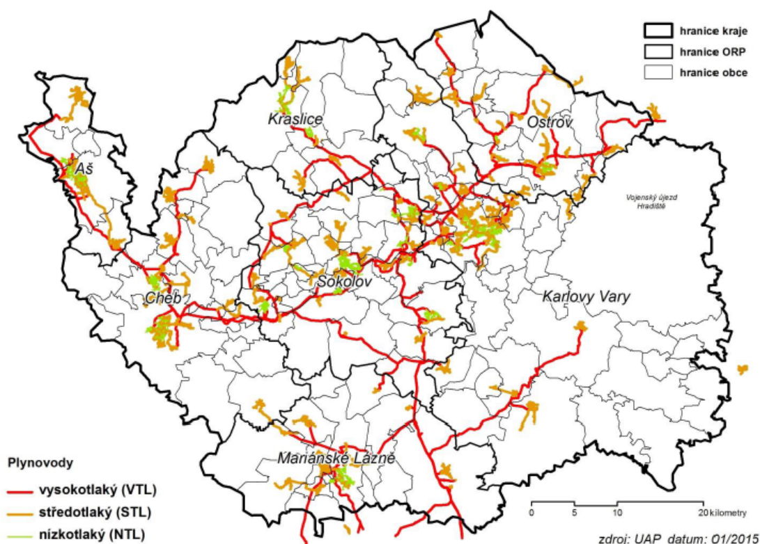
Obrázek 20 Síť plynovodů Karlovarského kraje (stav roku 2015)
