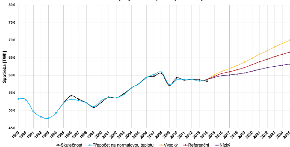
Graf 51 Předpokládané scénáře vývoje spotřeby elektřiny v ČR
