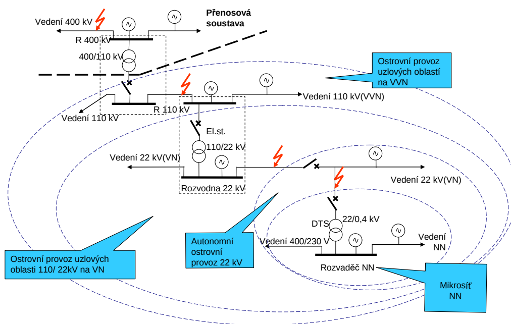
Obrázek 38 Možnosti ostrovního provozu v distribuční soustavě
