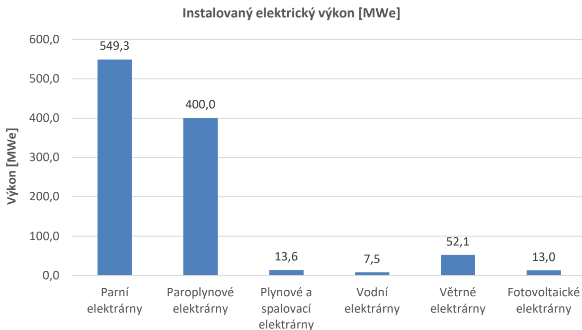
Graf 41 Instalovaný elektrický výkon dle technologie elektrárny
