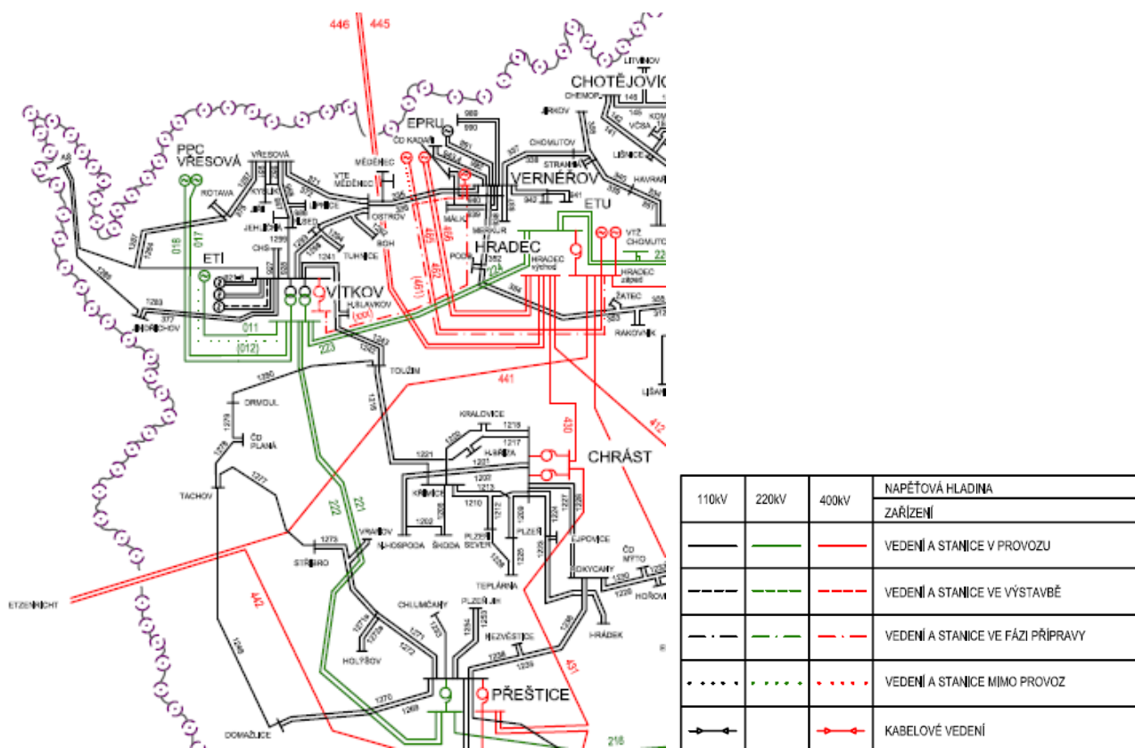
Obrázek 34 Elektrizační soustava na území Karlovarského kraje
