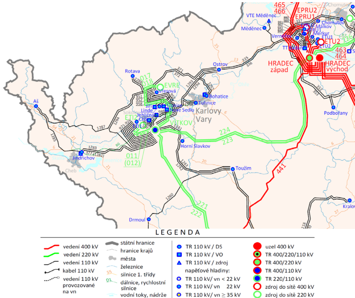
Obrázek 17 Schéma sítí 400, 220 a 110 kV v oblasti Karlovarského kraje vč. návaznosti za hranici kraje
