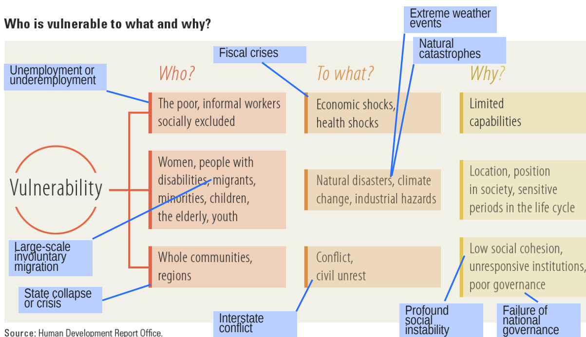
Obrázek 31 Přiřazení globálních rizik k mechanismu působení faktorů zranitelnosti
