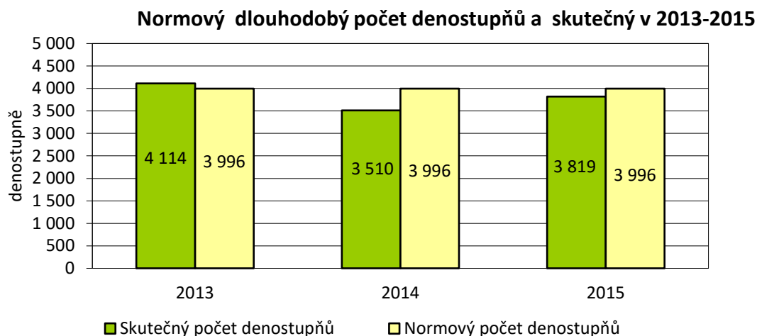
Graf 82 Porovnání klimatických údajů roku 2014 s dlouhodobým průměrem, denostupně
