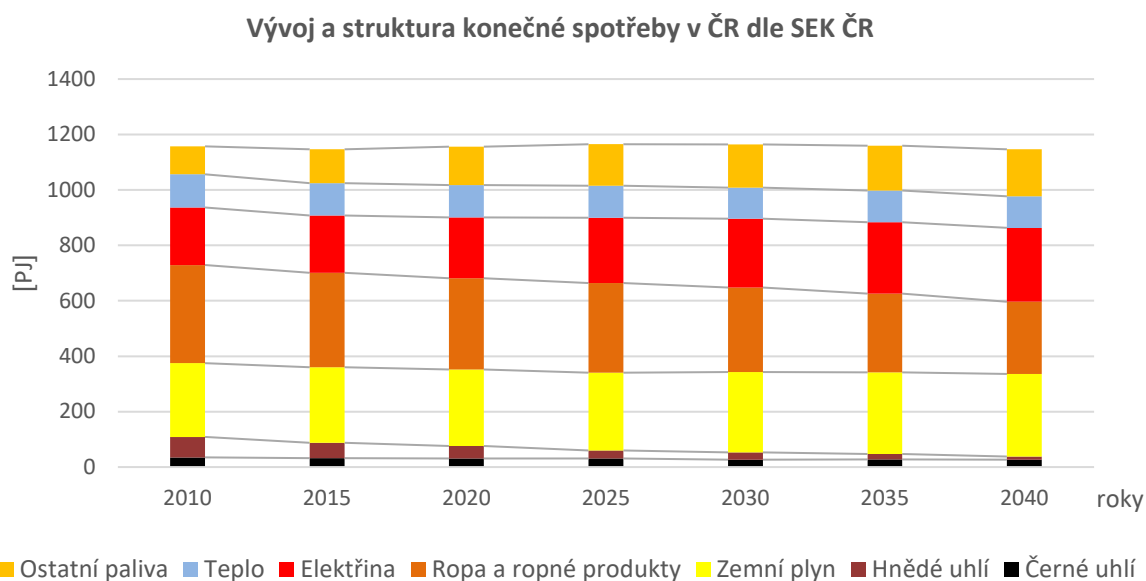
Graf 77 Vývoj a struktura konečné spotřeby energie v ČR dle (SEK)
